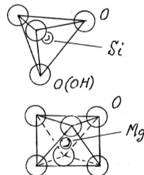
в — двуслойный пакет сеток [\text{SiO}_4]_{\infty} и [\text{Mg}(\text{OH})_6]_{\infty}
